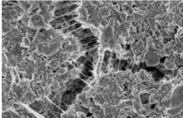
شکل ۸: نانو لوله های کربنی در ماتریس سیمان
