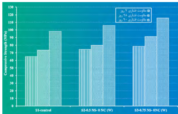
شکل ۳: اثر نانوسیلیکا بر مقاومت فشاری
