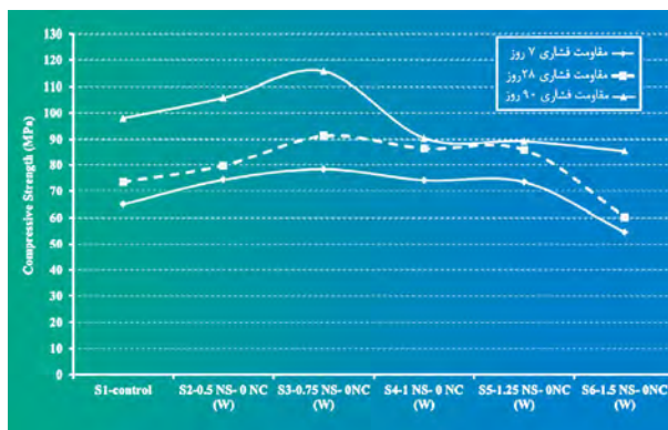
شکل ۵: درصد بهینه نانوسیلیکا برای مقاومت فشاری
