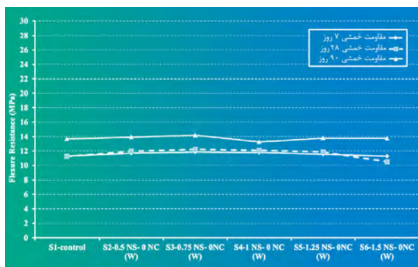
شکل ۶: درصد بهینه نانوسیلیکا برای مقاومت خمشی
