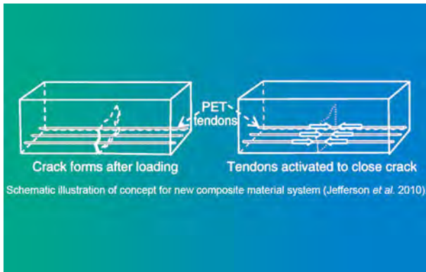
شکل ۰۱: سیستم خودترمیمی ارائه شده توسط Jefferson
