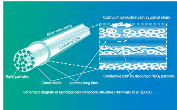
شکل ۱۱: دیاگرام شماتیک ساختار کامپوزیت شناساگر، ارائه شده توسط Nishiwaki
