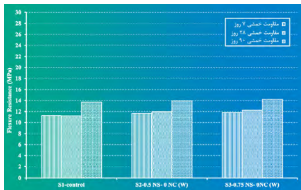
شکل ۴: اثر نانوسیلیکا بر مقاومت خمشی
