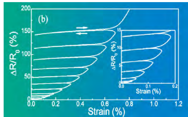
شکل ۲۱: ارتباط بین کرنش و نسبت تغییر مقاومت در حسگر پایش کننده کرنش، تحت بار کششی دوره ای
